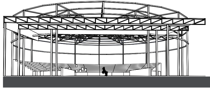
CORTE 1-1'
